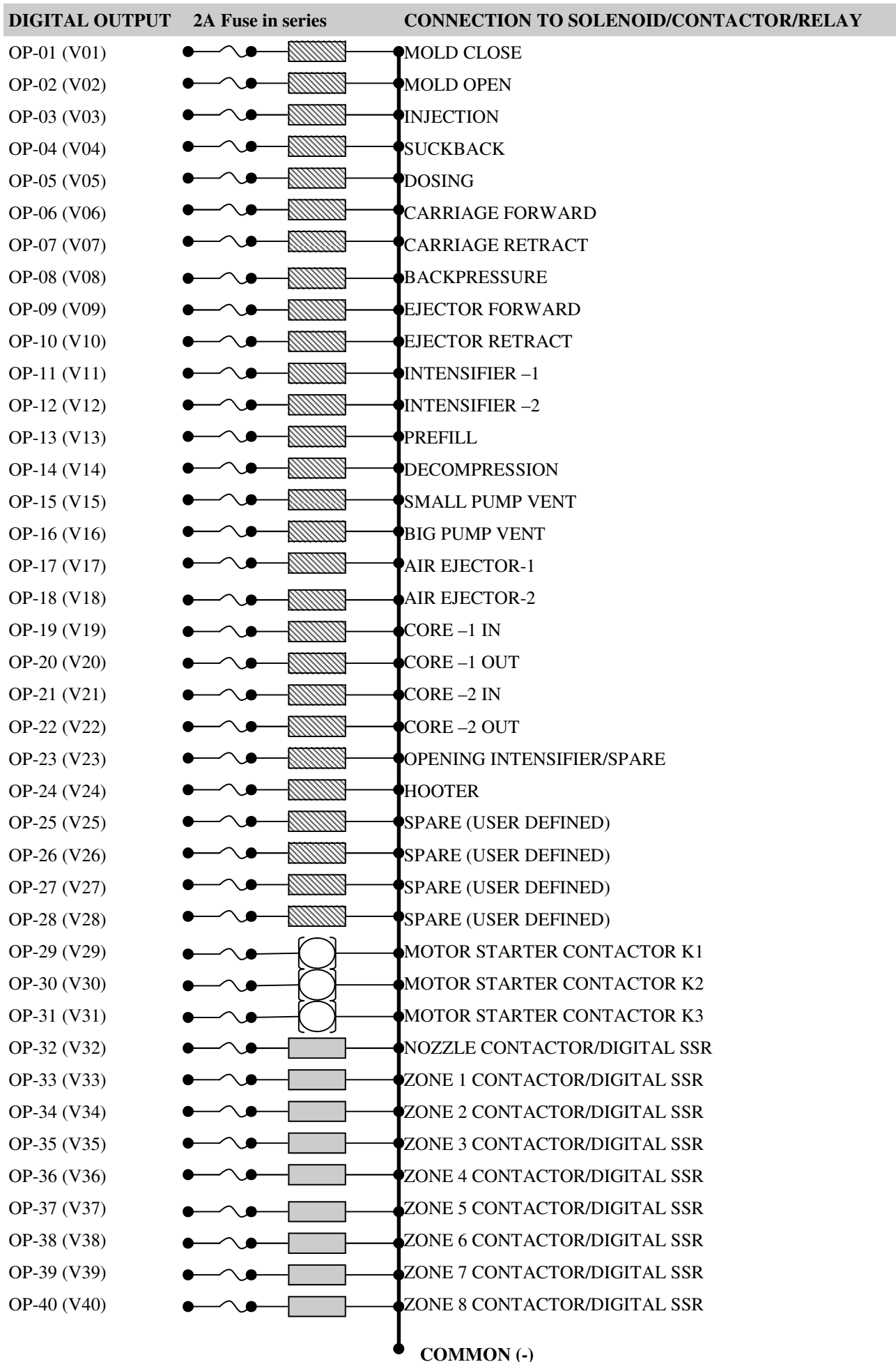
DIGITAL OUTPUTS (1-40) WIRING SCHEMATIC
